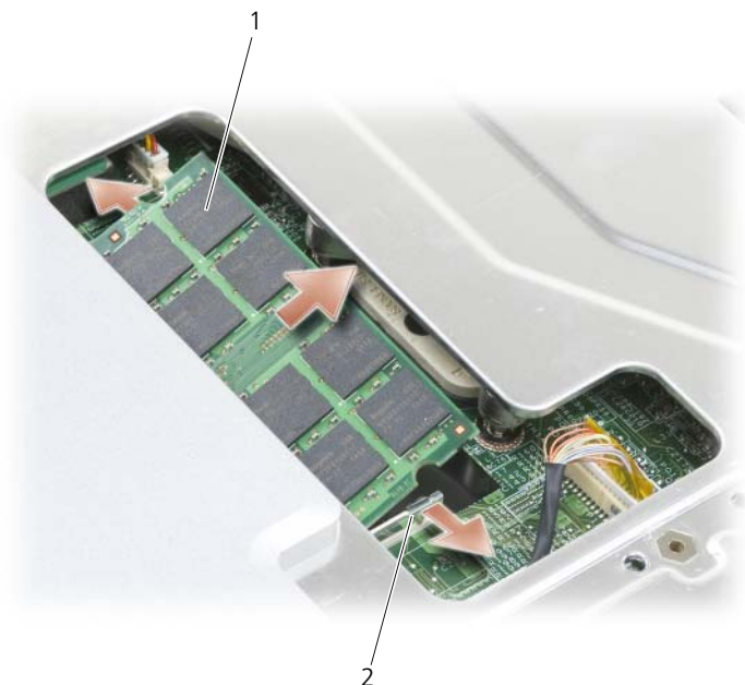
1 メモリモジュール (DIMM A) 2 固定クリップ (2)
